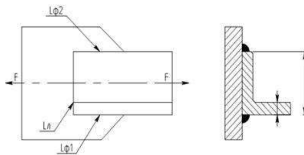
Рис. 4. Уголок, приваренный к косынке
