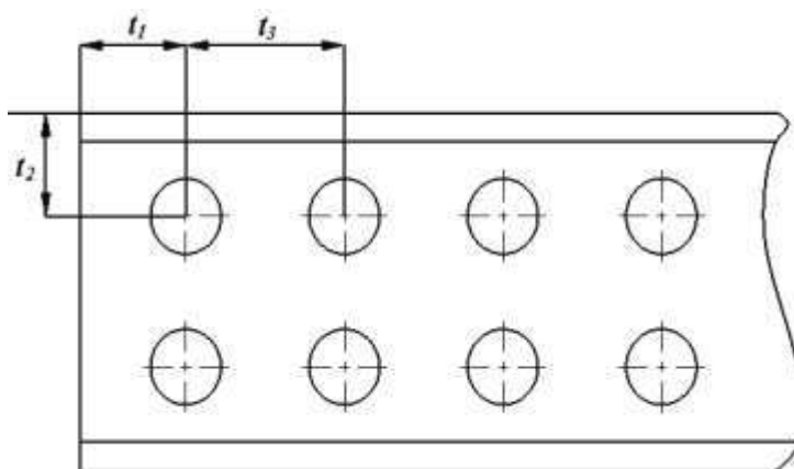
Рис. 6. Расстановка сварочных точек
