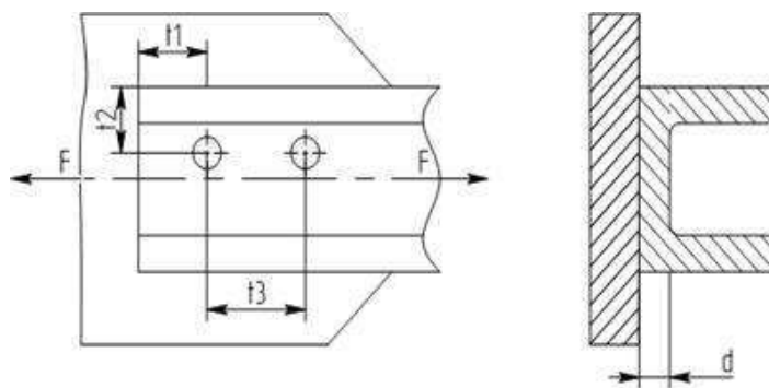
Рис. 5. Швеллер, приваренный к косынке точечной сваркой
