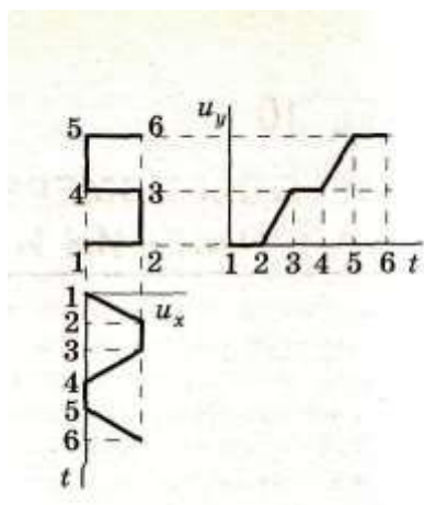
Рисунок 7 – Функции u_y(t) и u_x(t) для получения на экране цифры 5 по шрифту Бергера
