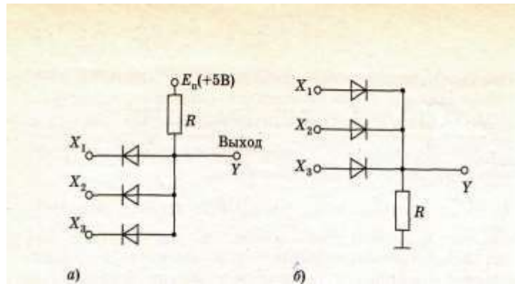
Рисунок 11 – Схемы диодных трехходовых элементов
