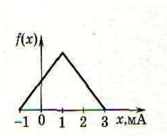
Рисунок 1 – Треугольное распределение
