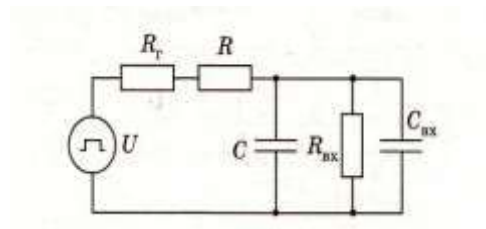
Рисунок 5 – Эквивалентная схема измерения u_c(t)
