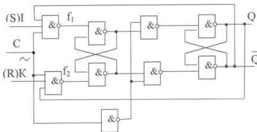
Рис. 4 Схема JK-триггера
