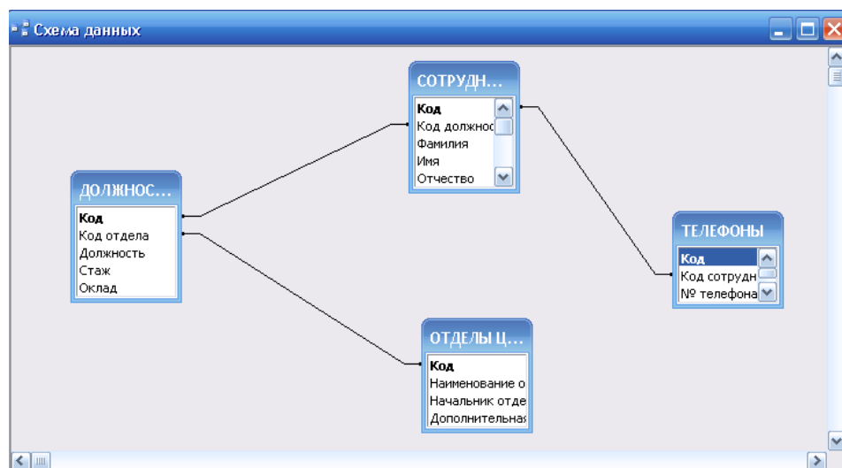
Рисунок 3 – Схема данных
